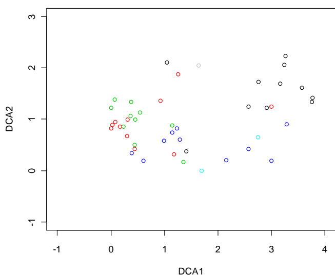
3-расм. 2010/11 йй. ўлат ва кўзилаш жойлари учун истисно қилинган трендли таҳлил асосида ординация. Нукталар билан алоҳида квадратлар кўрсатилган, ранг билан турли участкалар ажратилган: 2010 й. кўзилаш зонаси (қора), 2011 й. кўзилаш зонаси (кўк), 2010 й. ўлат зонаси (яшил) ва 2011 й. ўлат зонаси (қизил). бошқа рангли нукталар таркиби бир хил бўлган кўп сонли квадратларни кўрсатади.
