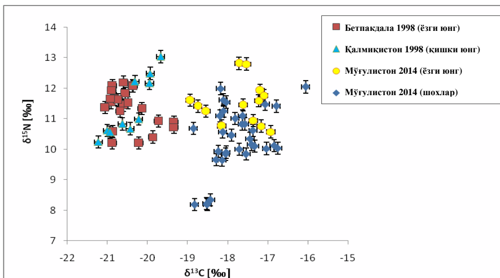
1-расм. Бетпақдала, Қалмиқистон ва Мўғулистон сайғоқларида \delta^{13}\text{C} ва \delta^{15}\text{N} қиймати. Мўғулистондан олинган намуналарда \delta^{13}\text{C} диапазони Бетпақдала ва Қалмиқистондаги популяцияларнинг шундай катталикларини қопламайди. (Такрорийлик: \delta^{13}\text{C} : \pm 0.1\% , \delta^{15}\text{N} : \pm 0.2\% .)
